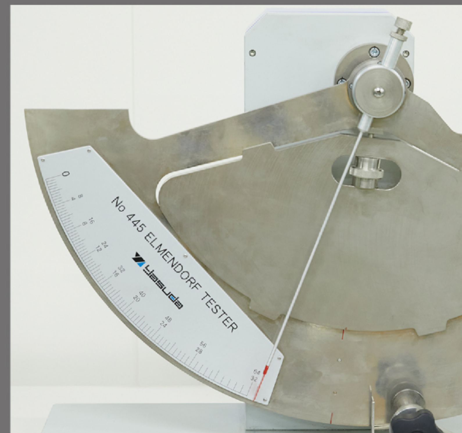
織布エルメンドルフ形引裂度試験機 (yasuda_No445)
